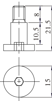
PC-30~40-M6
