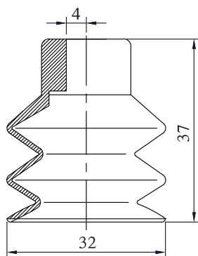
PCE-30
