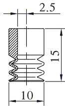
PCE-10
